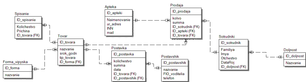
Рисунок 2. Физическая модель БД для автоматизации учета управления медикаментами и персоналом
