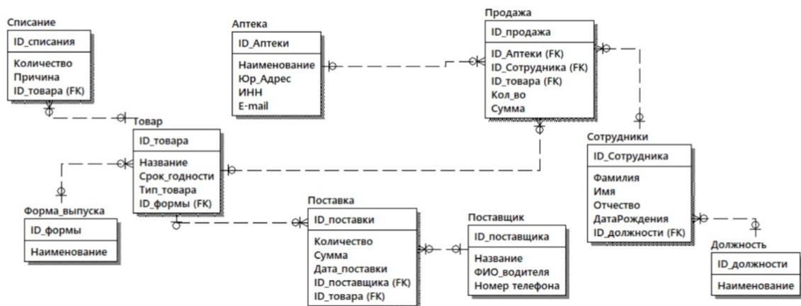
Рисунок 1. Логическая модель БД для автоматизации учета управления медикаментами и персоналом
